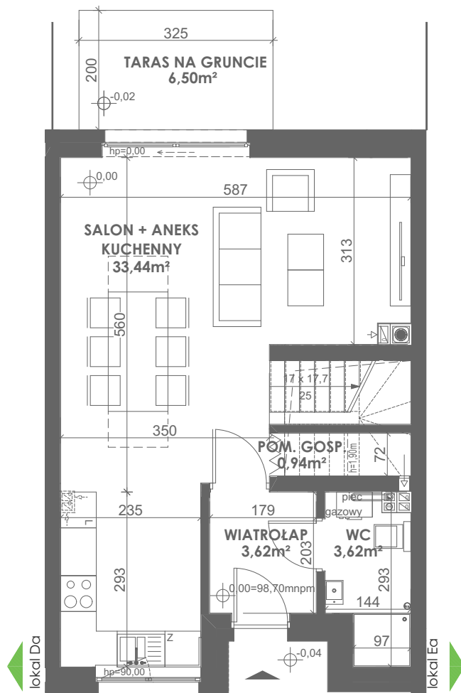
RZUT PARTERU
