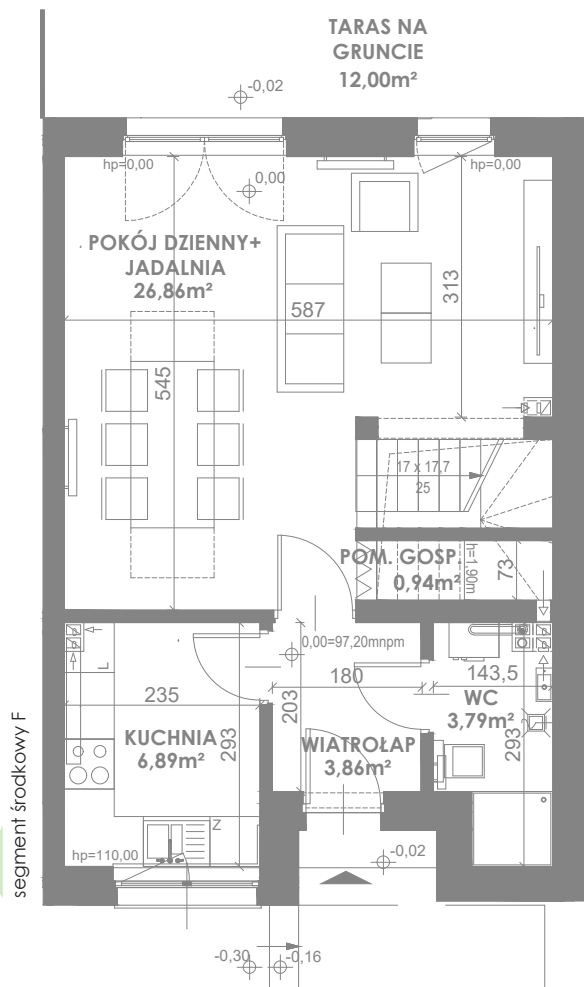
RZUT PARTERU
