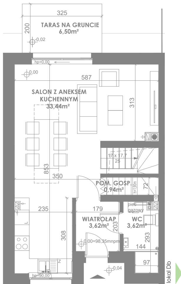
RZUT PARTERU
