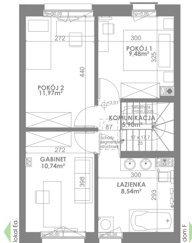
RZUT PIĘTRA
