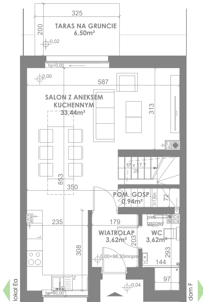
RZUT PARTERU
