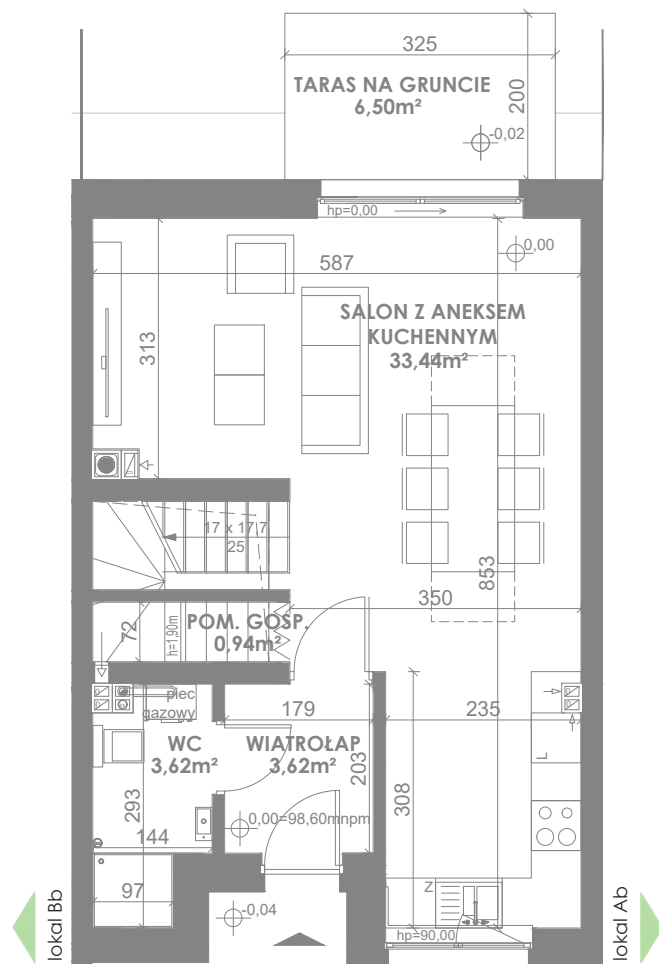
RZUT PARTERU
