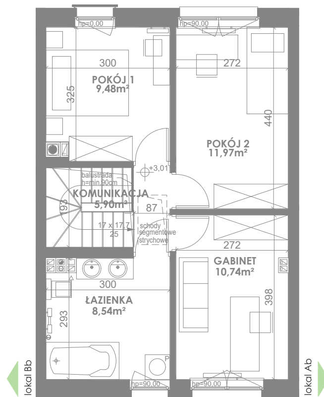
RZUT PIĘTRA
