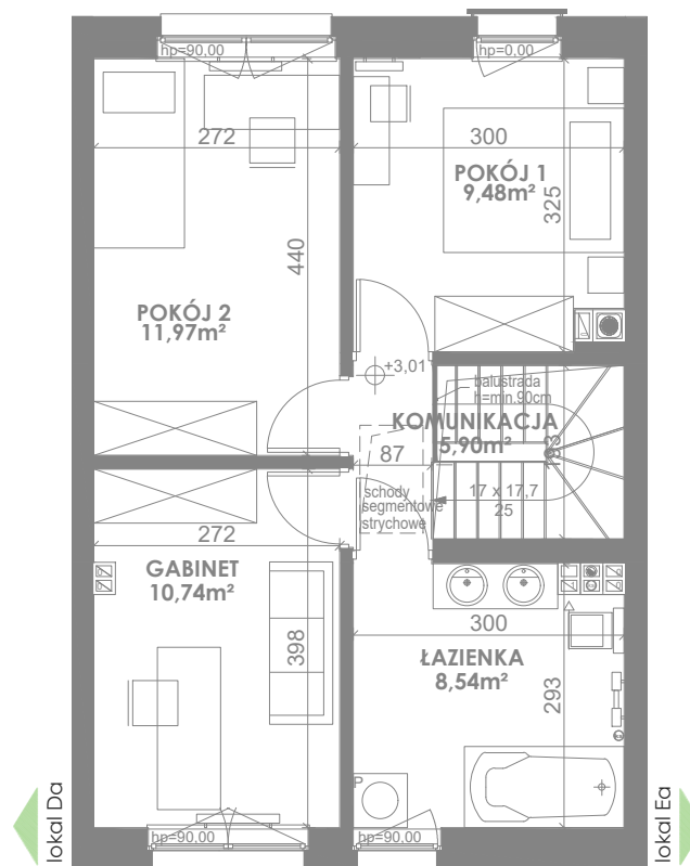
RZUT PIĘTRA
