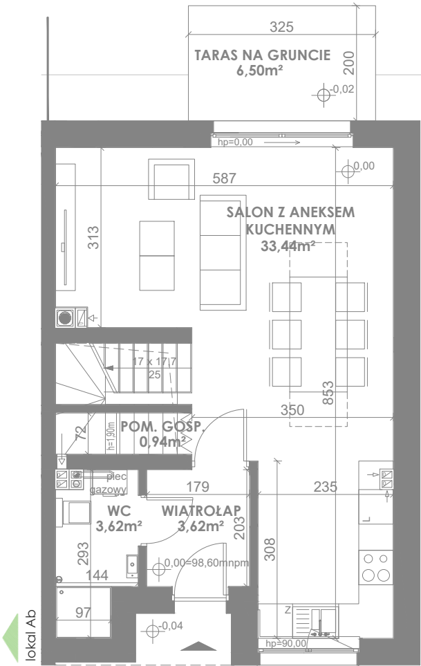
RZUT PARTERU
