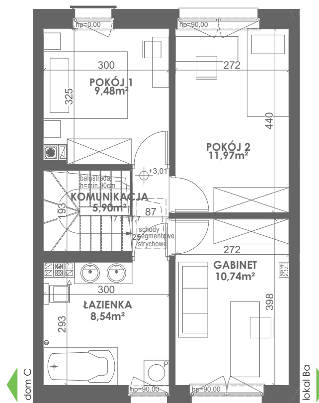
RZUT PIĘTRA
