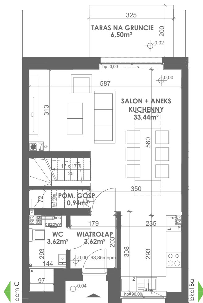
RZUT PARTERU
