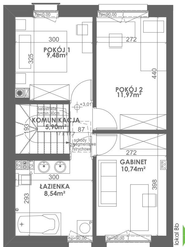
RZUT PIĘTRA
