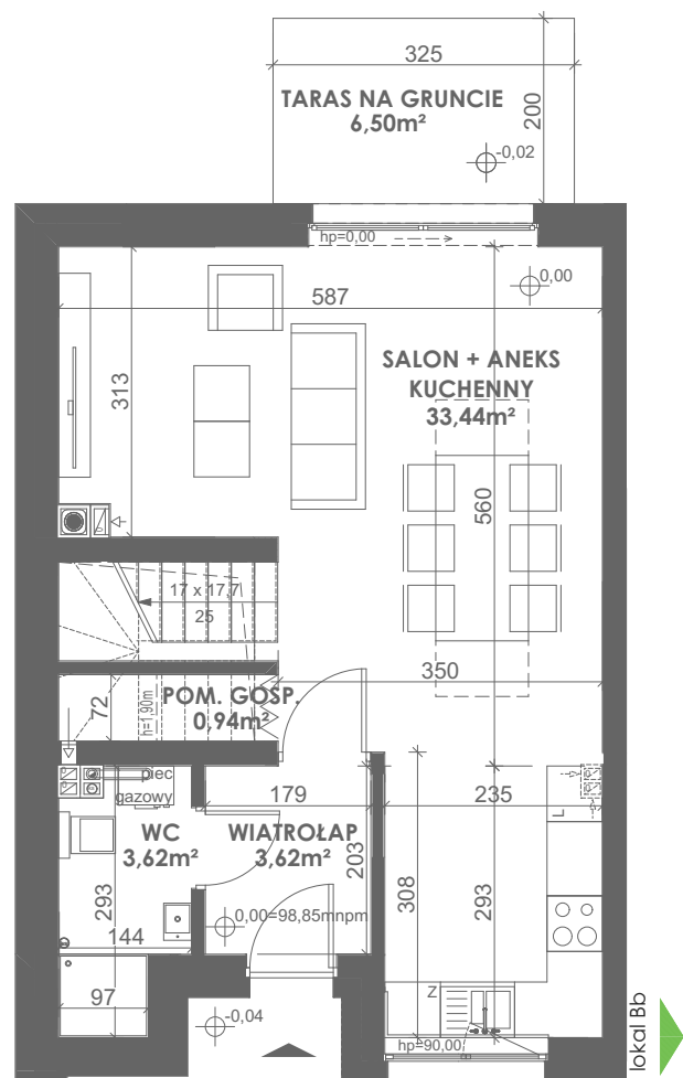
RZUT PARTERU
