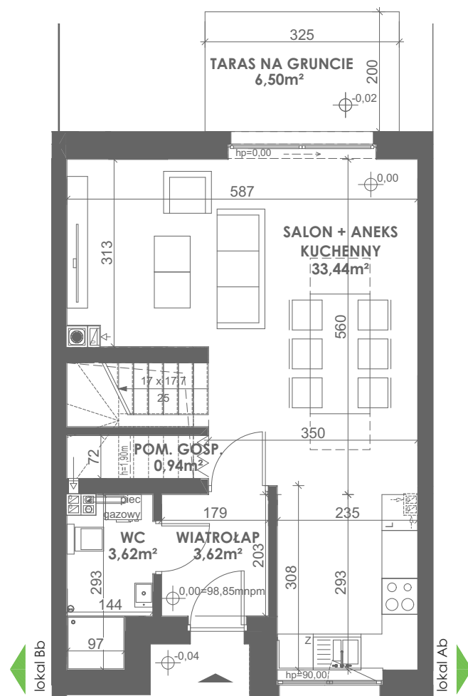
RZUT PARTERU
