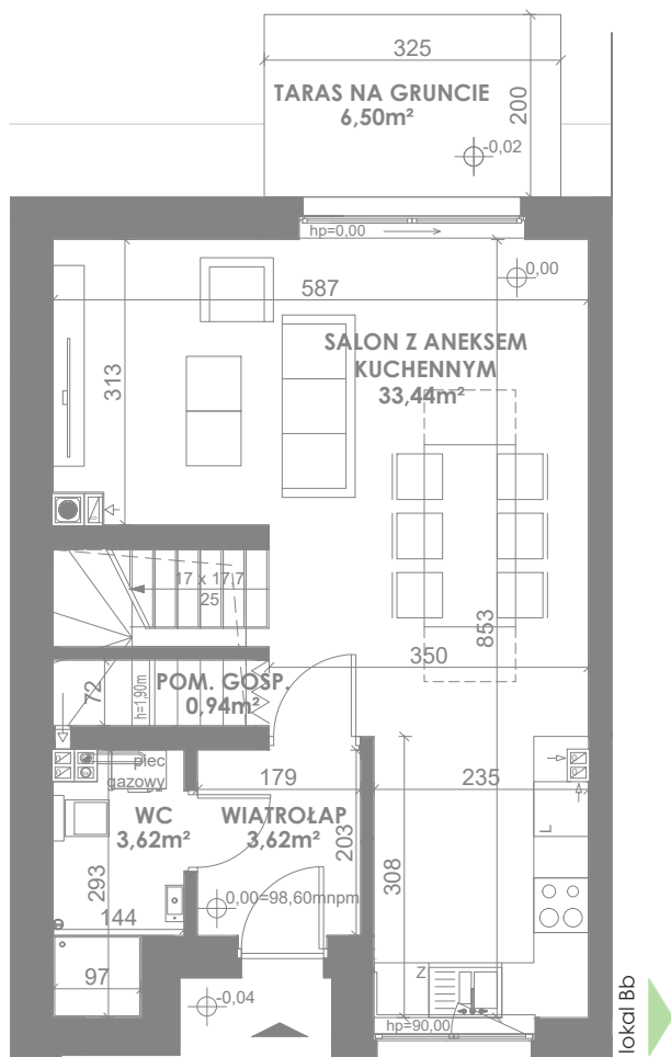
RZUT PARTERU
