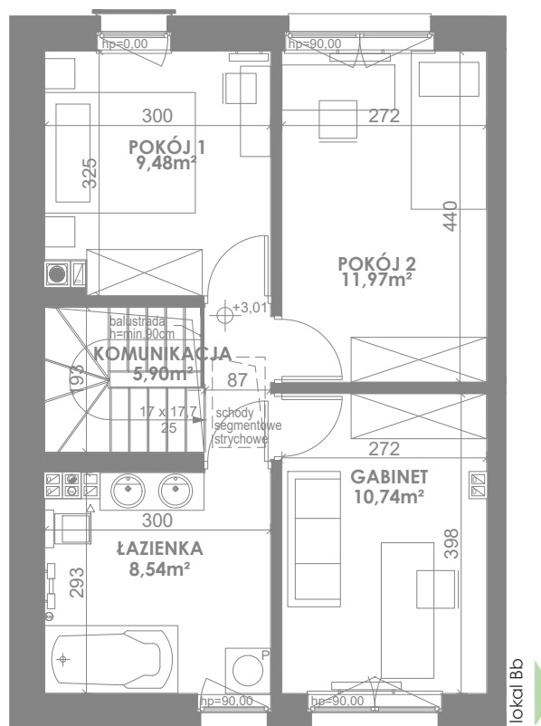
RZUT PIĘTRA
