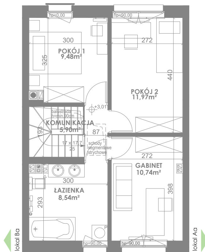
RZUT PIĘTRA
