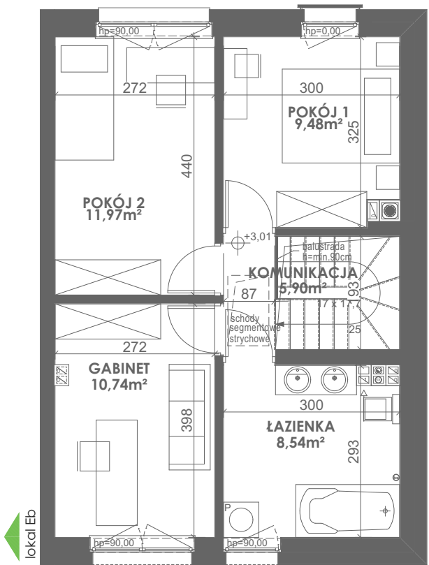
RZUT PIĘTRA
